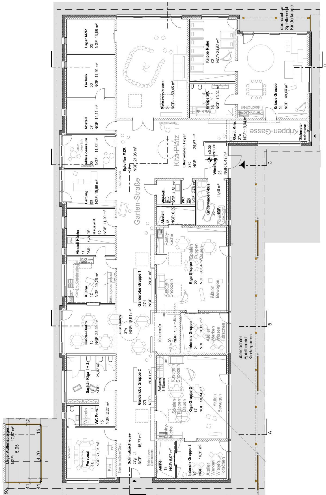
Abb. 1: Grundriss (selbst erstellt)
